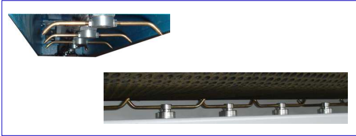
Soplador rotativo de limpieza paneles y tapete de transporte Soffiatore rotatico per pulizia pannelli e tappeto trasportatore
